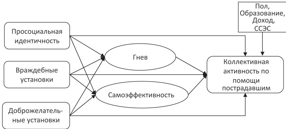
Рис. 1. Модель исследования
